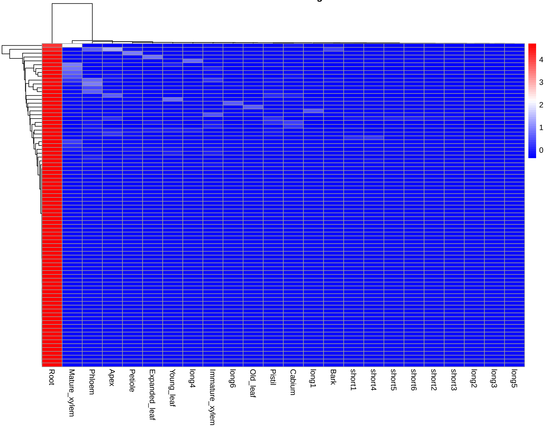
Module: brown - 84 genes
